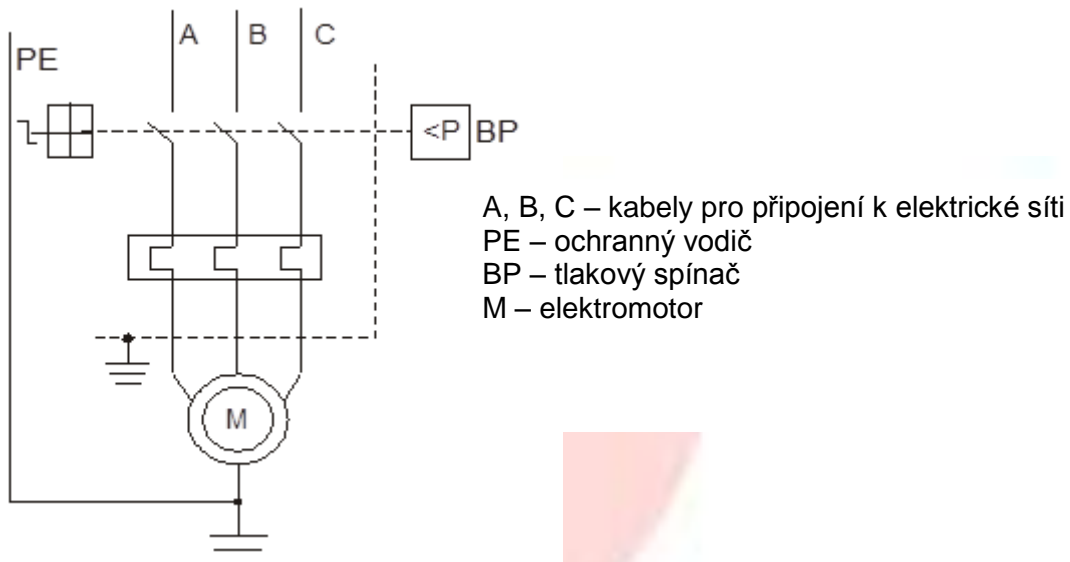
Obrázek A.1 – Schéma elektrických obvodů kompresorů C-50.LB24, C-100.LB24
