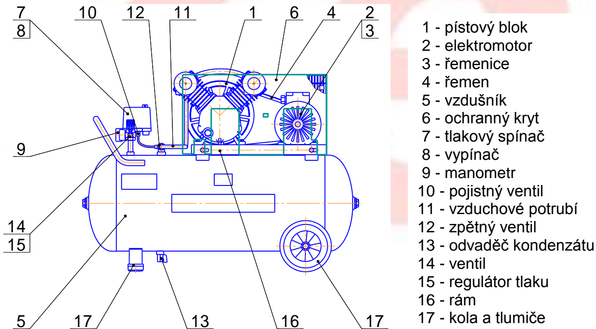
Obr. 8 - Celkový pohled na kompresor C-100.LB24A
