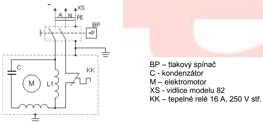
Obrázek A.2 – Schéma elektrických obvodů kompresorů C-50.LB24A, C-100.LB24A
