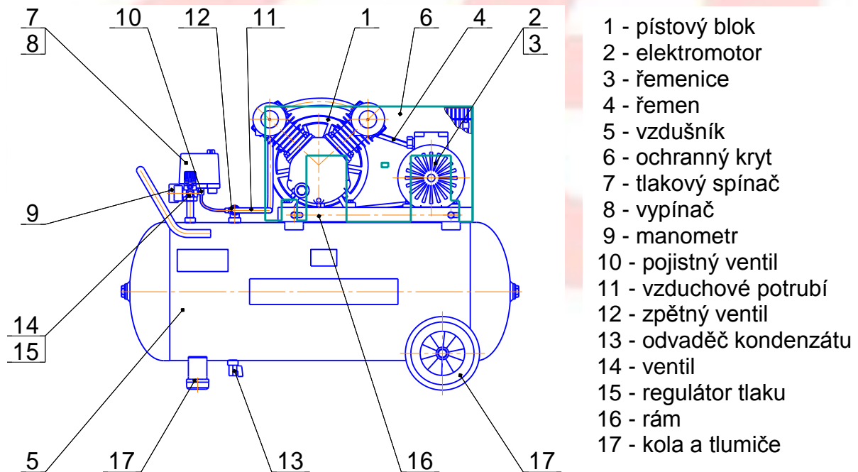
Obr. 5 - Celkový pohled na kompresor C-50.LB24
