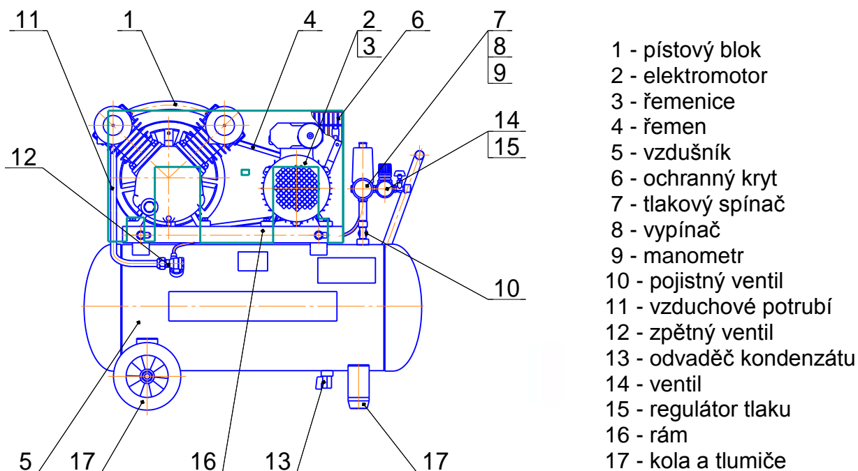
Obr. 7 - Celkový pohled na kompresor C-50.LB24A
